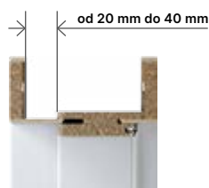
ZÁRUBNĚ S PRODLOUŽENÝM PEREM volitelně za příplatek
